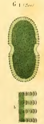
strigatum
