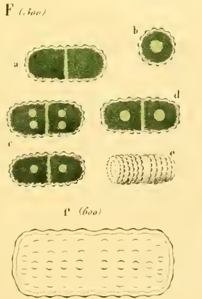
D. annulatum
