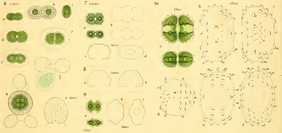
Eucastrum (Casmaticum)
