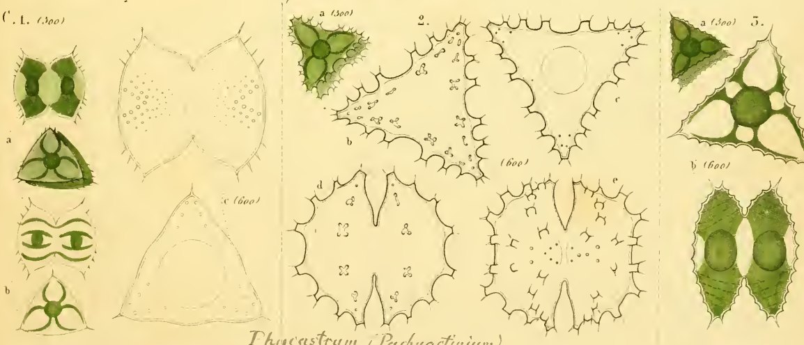
Phycostrium (Pachyactinium)
