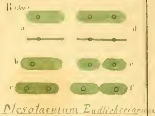
Mesotaenium Endlicherianum
