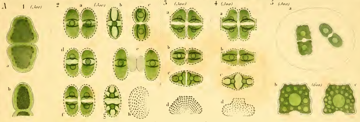
Eucastrum (Casmaticum)
