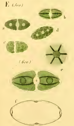
Dyosiphactium Regelii
