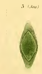
Euastrum (Microasterias)
