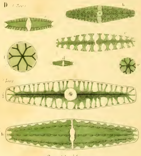
Cl. elegans
