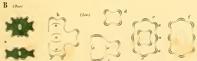
Eucastrum (Eucosmianum)
