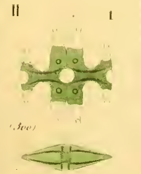
Dyosiphactium Regelii
