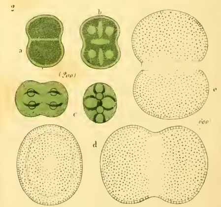
D. Meneghinianum
