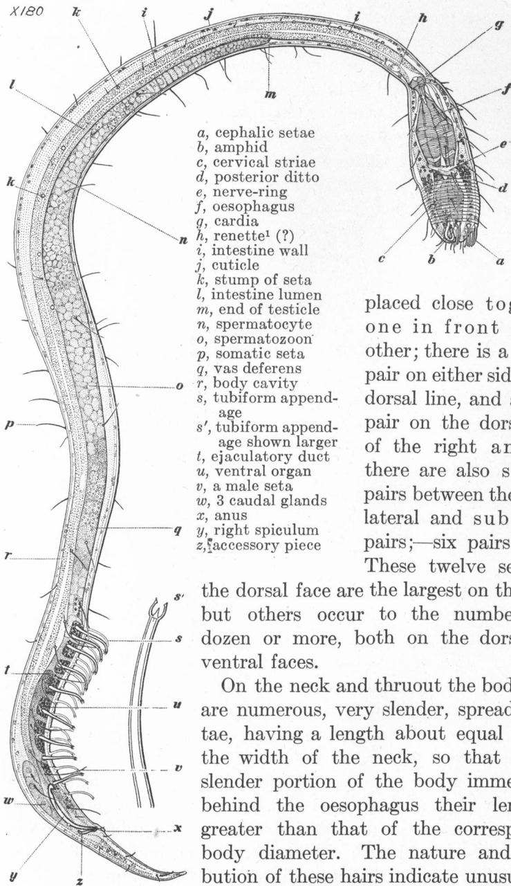
Fig. 1. Draconema cephalata
